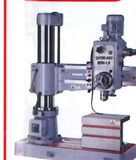
ラジアルボール盤 BRNシリーズ
