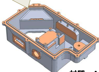
インバータケース W1000Xd1 (16000回転仕様)
