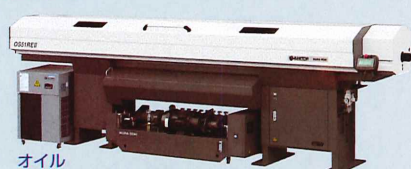
自動棒材供給機 OS51REII
